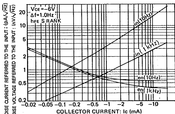
Fig.13 電圧性雑音電流性雑音—コレクタ電流特性
