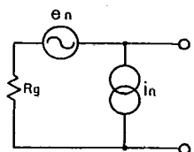
測定回路
