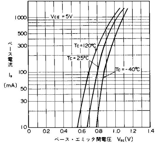
ベース入力特性 Base Input Characteristics
