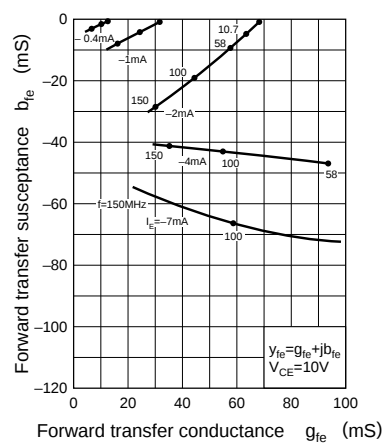
b_{fe} - g_{fe}
