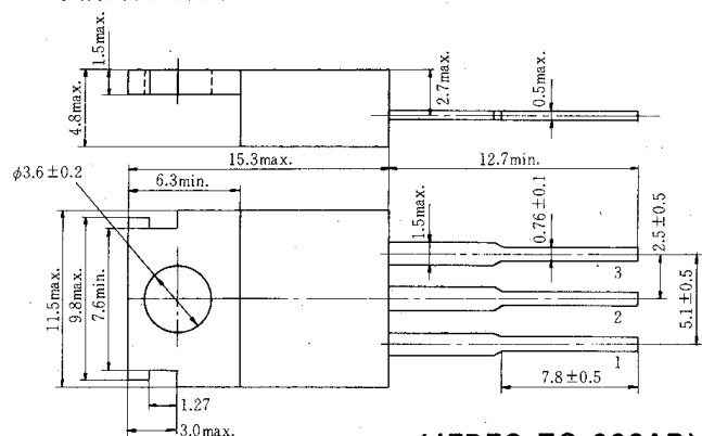
(JEDEC TO-220AB)
