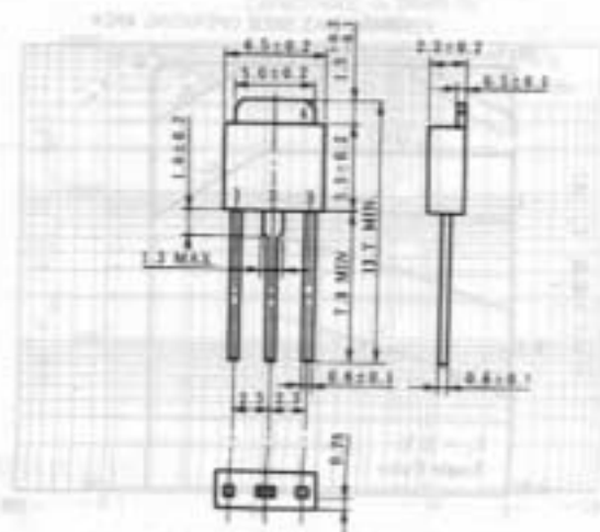
2SJ132外形図
