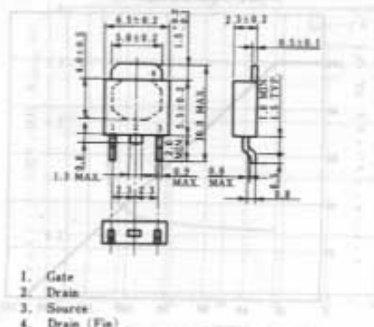
2SJ132-Z外形図
