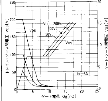
ゲートチャージ特性 Gate Charge Characteristics
