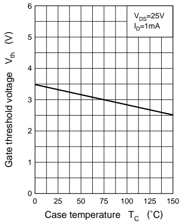
V_{th} - T_C
