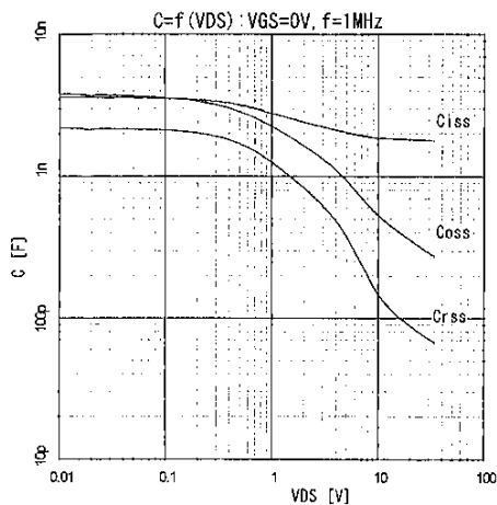
入力/出力帰還容量 Typical capacitances
