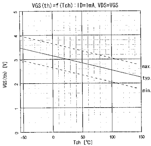
ゲートしきい値電圧 Gate threshold voltage
