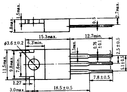
(JEDEC TO-220AB)
