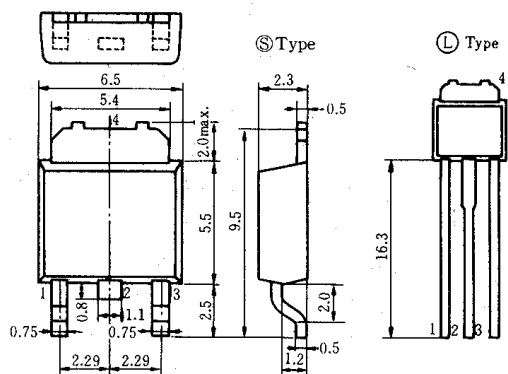
(DPAK)
