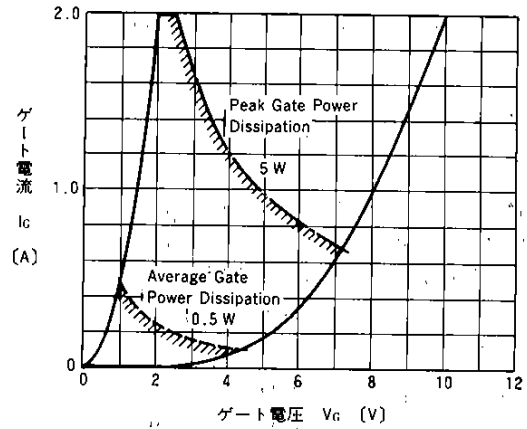
ゲート特性(ゲート損失) Gate Characteristics
