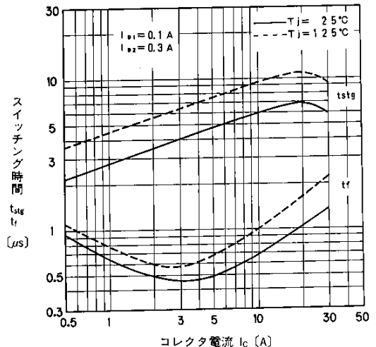
スイッチング時間 t_{sg} t_r コレクタ電流 I_c (A) スイッチング時間-コレクタ電流特性 Switching Time
