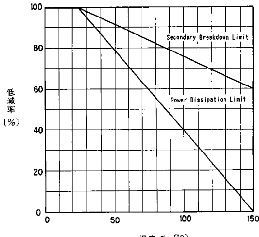
ケース温度 T_c (°C) ASO低減特性 ASO Derating
