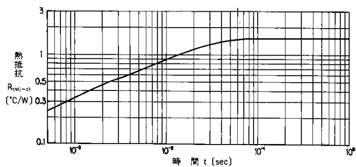
過渡熱抵抗(ダイオード)特性
