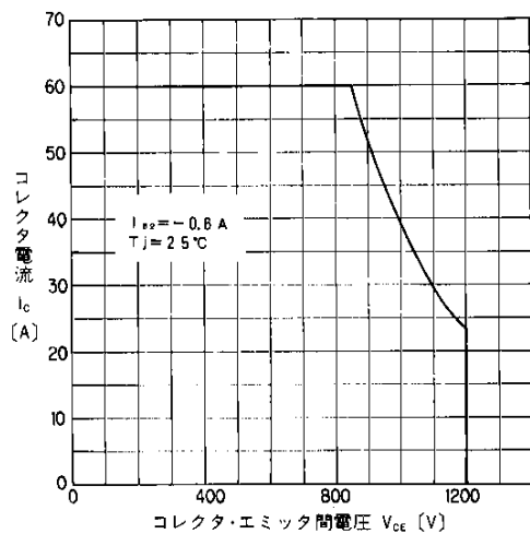
安全動作領域(逆バイアス)
