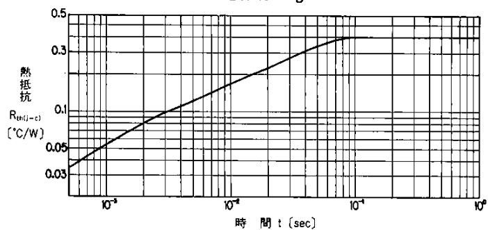
過渡熱抵抗(トランジスタ)特性
