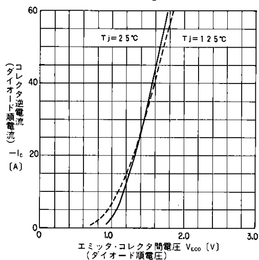
高速フリーホイーリングダイオード順電圧
