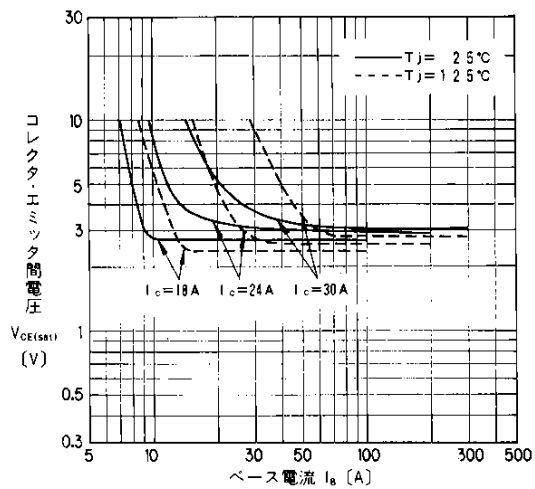
出力特性
