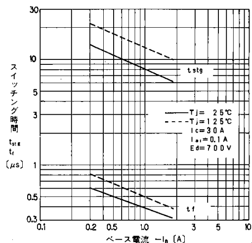
スイッチング時間—ベース電流特性
