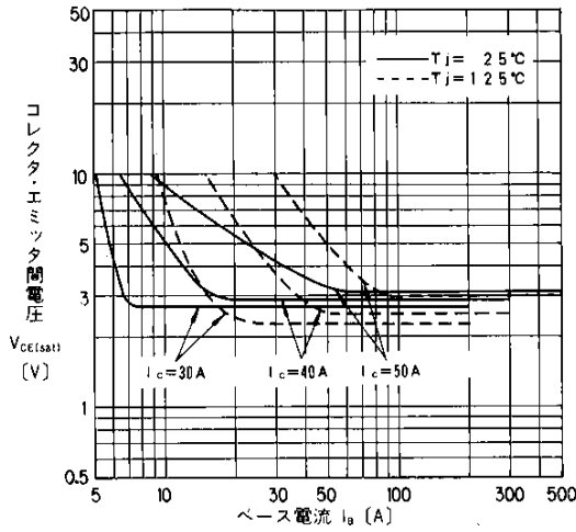
出力特性
