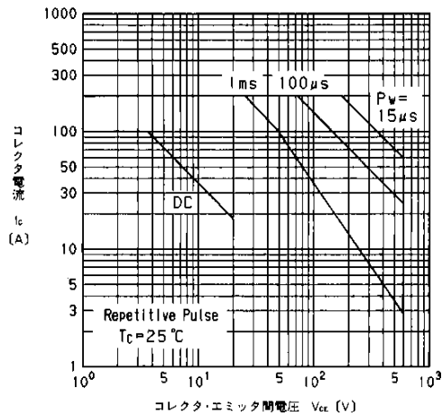
安全動作領域 (繰返し) Safe Operating Area
