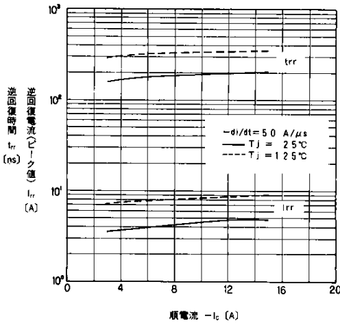
T_{rr} - I_c - T 特性 T_{rr} - I_c - T
