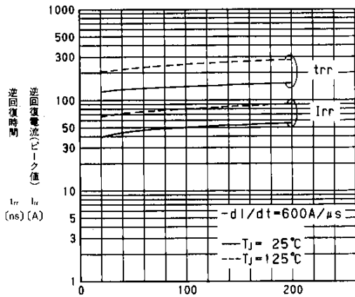
T_{rr} , I_{rr} - I_d 特性 T_{rr} , I_{rr} - I_d
