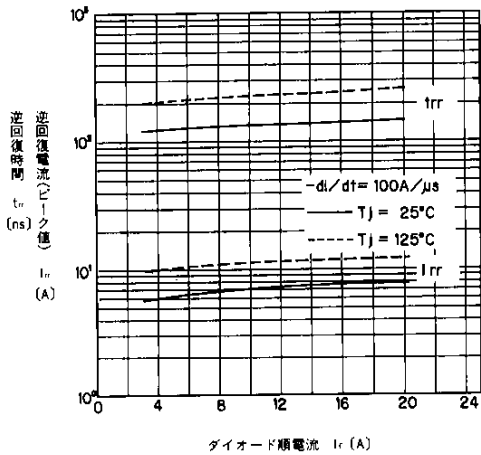
t_{rr} , I_{rr} - I_f 特性 T_{rr} , I_{rr} - I_f
