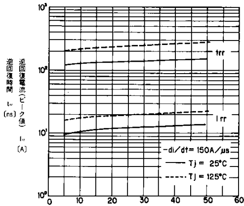
ダイオード順電流 I_{fr} (A) t_{rr} , I_{rr} - I_{fr} 特性 T_{rr} , I_{rr} - I_{fr}
