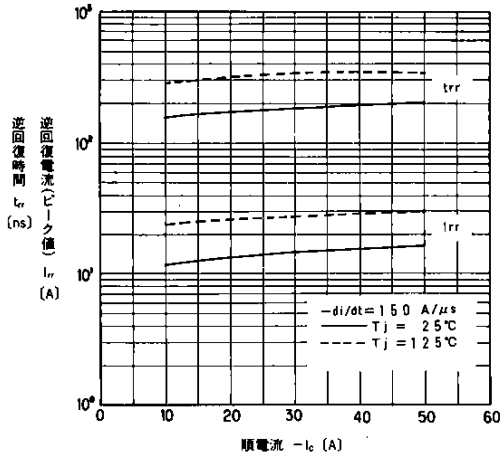
T_{rr} , I_{tr} - I_f 特性 T_{rr} , I_{tr} - I_f
