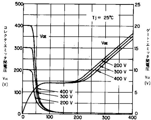
ダイナミック入力特性 Dynamic Input Characteristic
