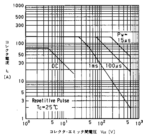
安全動作領域 (繰返し) Safe Operating Area
