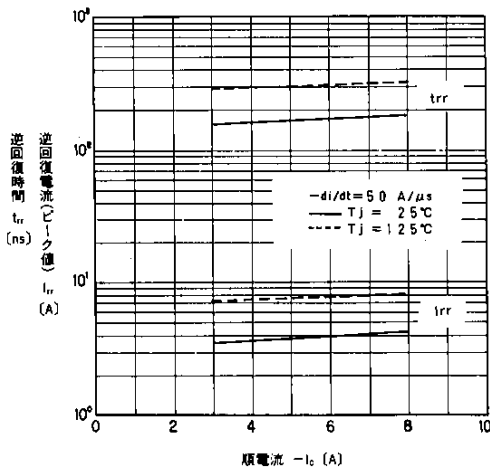
T_{rr} , t_{rr} - I_c 特性 T_{rr} , t_{rr} - I_c
