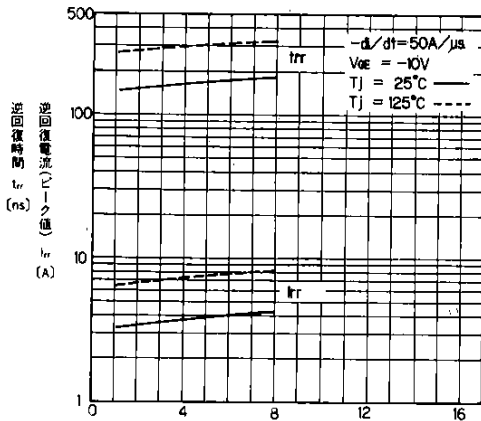
T_{rr} , I_r - I_f 特性 T_{rr} , I_r - I_f
