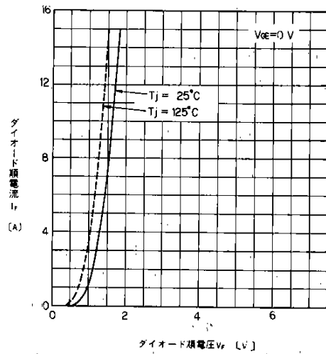
高速フリーホイリングダイオード順電圧特性 Forward Voltage of Free Wheeling Diode
