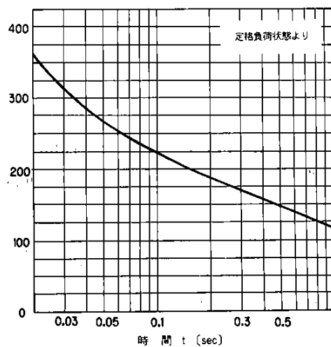
サージ電流 Surge Current
