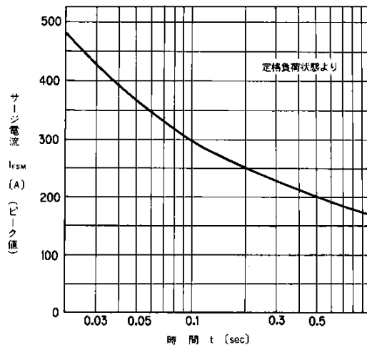
サージ電流 Surge Current
