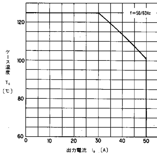
出力電流 - ケース温度 Output Current - Case Temperature
