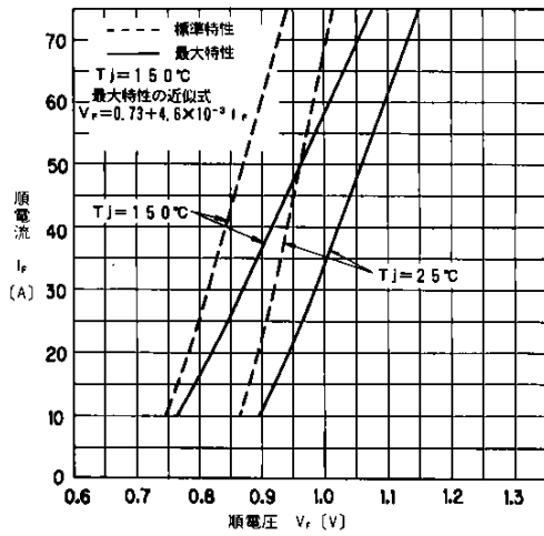
順電圧特性 Forward Characteristics
