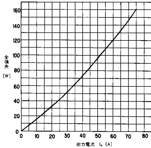
出力電流 - 全損失 Output Current - Total Loss
