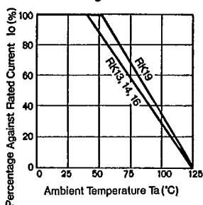
Io - Ta Deratings
