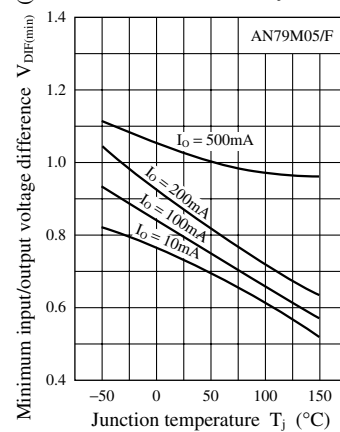
V_{DIF(min)} - T_j
