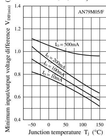
V_{DIF(min)} - T_j
