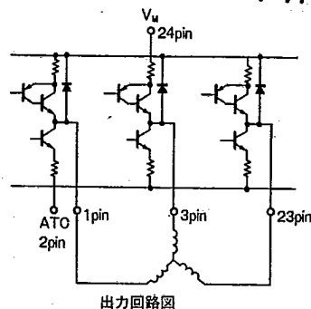
出力回路図
