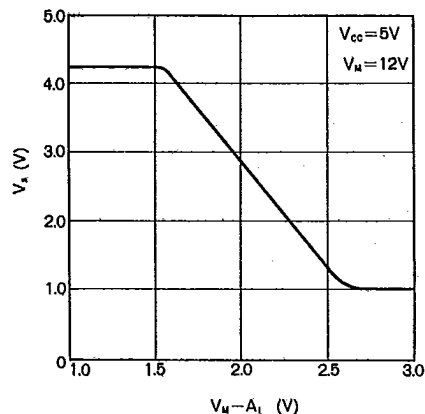
Fig.9 飽和検出力- V_M ・出力端子間電圧特性
