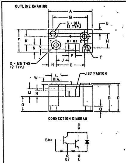
500-600-700 Volt D67DE Outline Drawing
