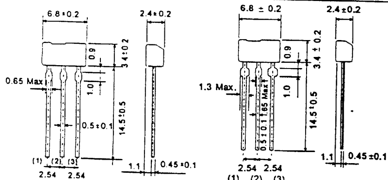
FTL(TL2 Style) Package
