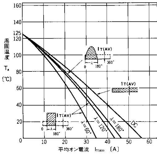
平均オン電流—周囲温度 (冷却体AH01-12, 自冷)
