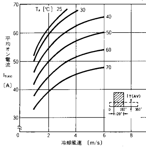
平均オン電流—冷却風速 (方形波120°導通, 冷却体AH02-12)
