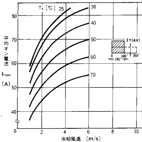
平均オン電流—冷却風速 (方形波180°導通, 冷却体AH02-12)
