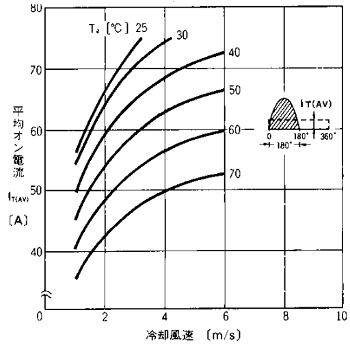
平均オン電流—冷却風速 (正弦波180°導通, 冷却体AH02-12)
