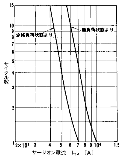
サージオン電流
