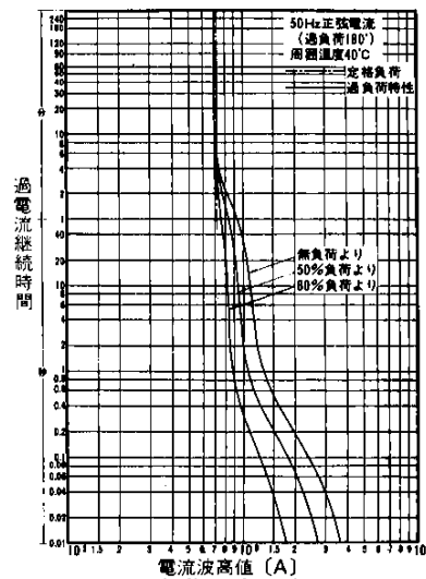
過負荷電流—時間 (冷却体AL01-24, 風冷6m/s)
