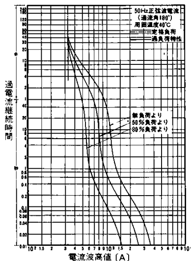
過負荷電流—時間 (冷却体AL01-24, 自冷)
