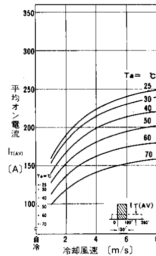
平均オン電流—冷却風速 (方形波120°導通, 冷却体AL01-24)
