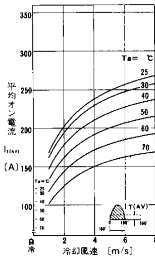
平均オン電流—冷却風速 (正弦波180°導通, 冷却体AL01-24)
