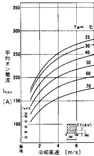
平均オン電流—冷却風速 (方形波180°導通, 冷却体AL01-24)
