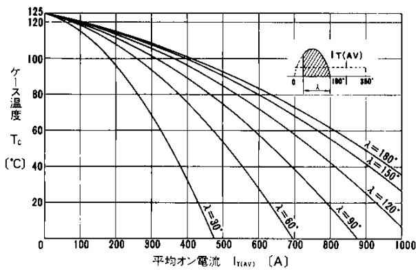
平均オン電流—ケース温度(正弦波電流)
