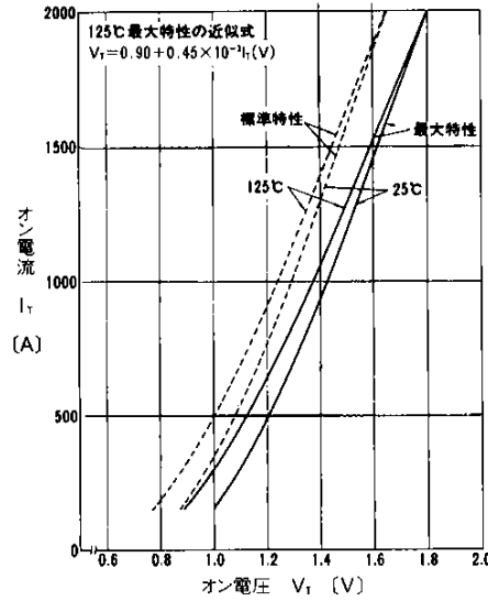
オン電圧特性
