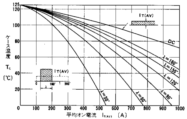
平均オン電流—ケース温度(方形波電流)
