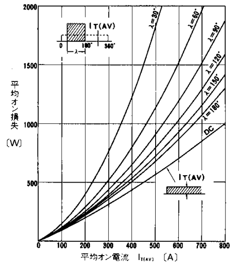
平均オン損失(方形波電流)
