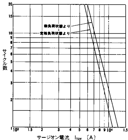
サージオン電流
