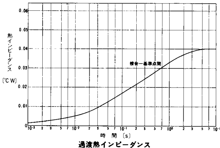
過渡熱インピーダンス
