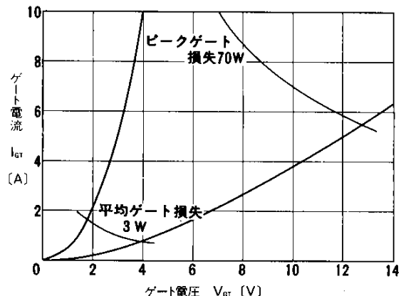
ゲート特性
