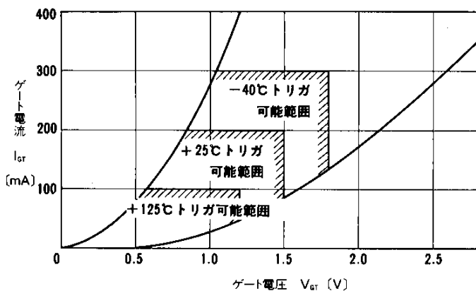
ゲートトリガ特性
