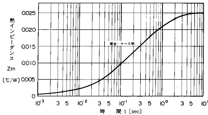
過渡熱インピーダンス
