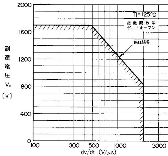
臨界オフ電圧上昇率 dv/dt Characteristics
