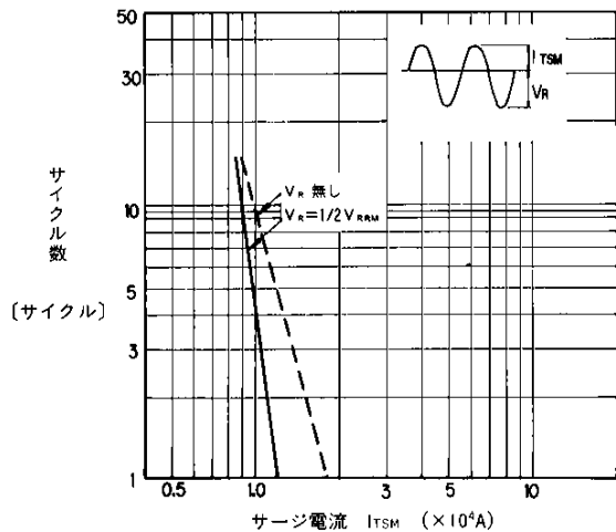
サージ電流耐量 Surge Capability
