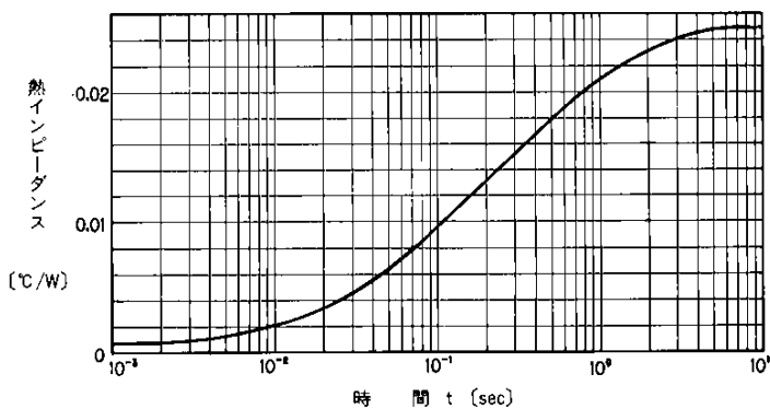
過渡熱インピーダンス
