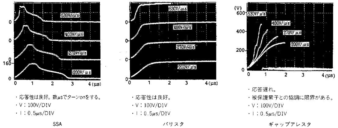
図8-1 dv/dtによるV cl の依存性と応答性
