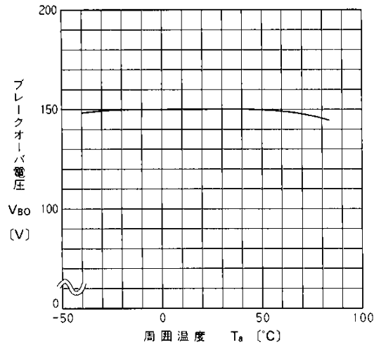
ブレイクオーバー電圧-温度依存性(代表特性) Breakover Voltage
