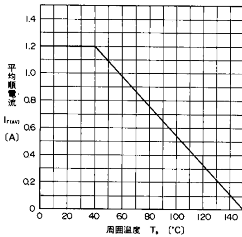
平均順電流一周囲温度特性 Current Derating ( I_{F(AV)}-T_a )
