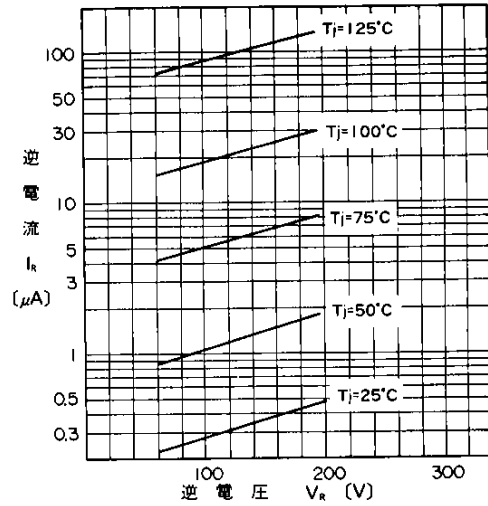
逆特性 (代表特性) Reverse Characteristics
