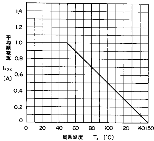
平均順電流一周囲温度特性 Current Derating ( I_{F(AV)}-T_a )
