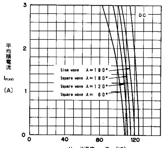
平均順電流—リード温度特性 Current Derating ( I_{F(AV)}-T_2 )
