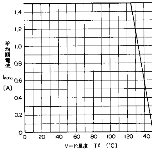
平均順電流-リード温度特性 Current Derating ( I_{F(AV)}-T_l )
