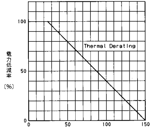
ケース温度 T_c (°C) 電力低減特性 P_C Derating
