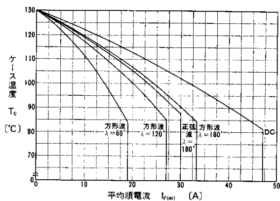
平均順電流—ケース温度(50Hz)
