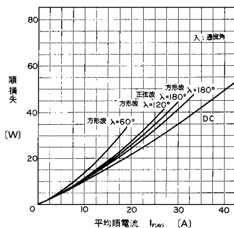
順損失(50Hz)
