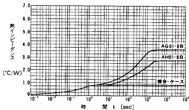
過渡熱インピーダンス
