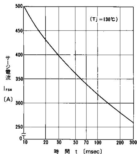
サージ電流 (50Hz正弦波)
