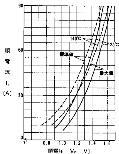
順特性
