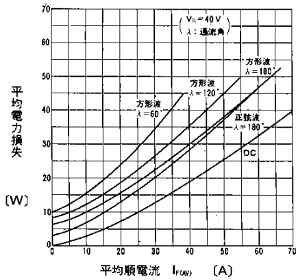
平均電力損失
