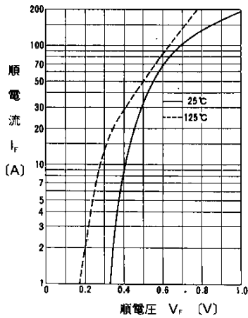
順特性
