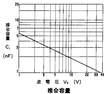
接合容量
