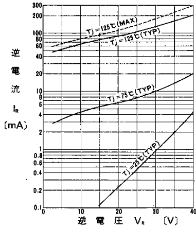
逆特性
