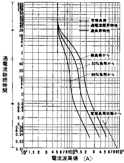
過負荷電流—時間 (冷却体AL01-24) 自冷 50Hz正弦波電流(通流角180°)
