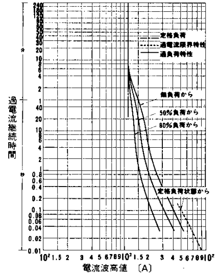
過負荷電流—時間 (冷却体AL01-24) 風冷6m/s 50Hz正弦波電流(通流角180°)
